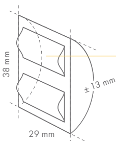
Cubito de KM Edge Peso: 10 g
